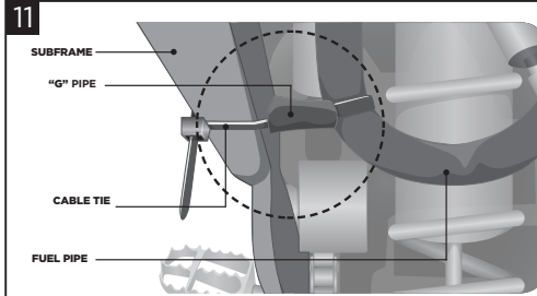
11 Fix the fuel pipe on the subframe (left side) with the plastic strap, use the "G PIPE" to separate the subframe from fuel pipe. Fissare con la fascetta il tubo benzina al telaio (lato sinistro) usando il "TUBO G" come distanziale.
