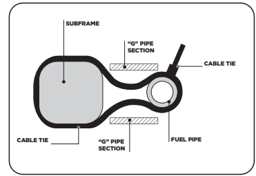
11 Fix the fuel pipe on the subframe (left side) with the plastic strap, use the "G PIPE" to separate the subframe from fuel pipe. Fissare con la fascetta il tubo benzina al telaio (lato sinistro) usando il "TUBO G" come distanziale.
