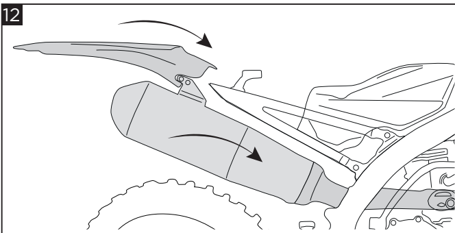
12 Mount the silencer and rear fender. Montare il silenziatore e il parafrangente posteriore.
