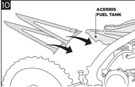
10 Remount the rear subframe. Rimontare il telaio posteriore.
