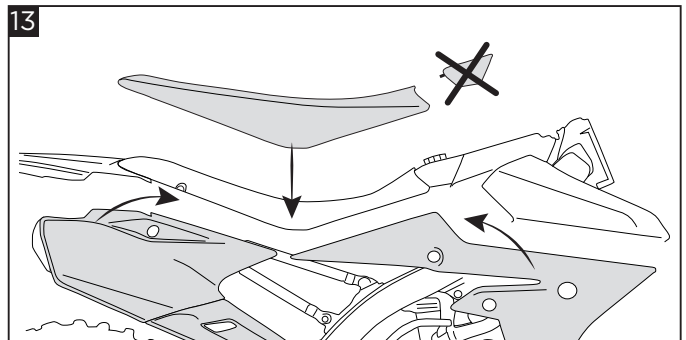
13 Mount plastics and the seat. Rimontare plastiche moto e sella.
